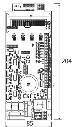
DIMENSIONI CN3-AT
