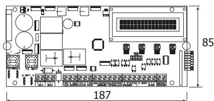
DIMENSIONI CN3-BT
